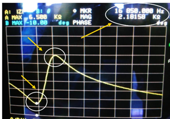
شکل 16 منحنی امپدانس الکتریکی برحسب فرکانس
