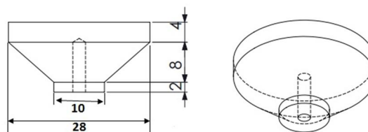
شکل 4 جرم سر آلومینیومی
