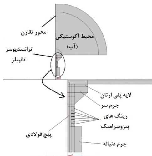
شکل 6 شکل شماتیک محیط آکوستیکی و ترانس‌دیوسر تانپیلز مدل شده در نرم‌افزار اجزاء محدود
