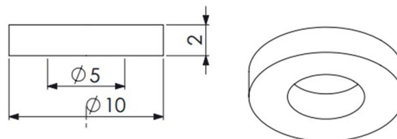
شکل 3 رینگ پیزوسرامیک مورد استفاده
