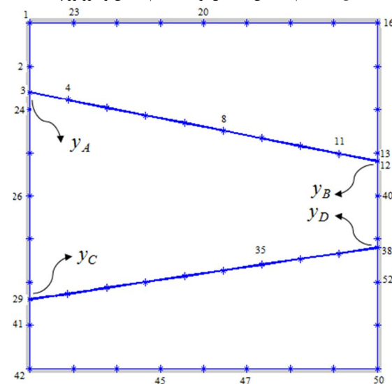
شکل 11 نحوه المان بندی و شماره گذاری گره‌ها
