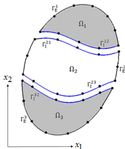
شکل 3 جسم الاستیک ناهمگن با سه زیر ناحیه در تماس
