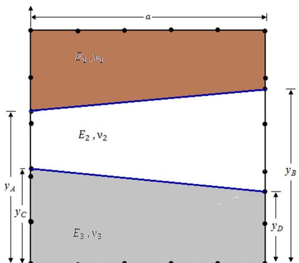
شکل 5 جسم الاستیک ناهمگن با سه زیر ناحیه در تماس
