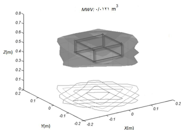
شکل 7 فضای کاری بیشینه (MWV) و بزرگترین مکعب قابل محاط شدن در آن
