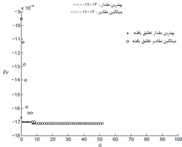
شکل 8 همگرایی نتایج بهینه‌یابی ساختار با فضای کاری بیشینه (MWV)
