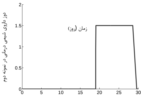
شکل 7 ورودی کنترلی (داروی شیمی درمانی)
