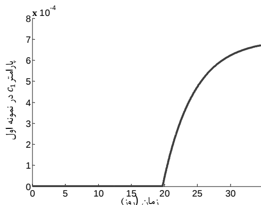
شکل 3 تغییرات پارامتر c_1 در طول دوره درمان
