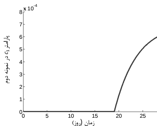
شکل 6 تغییرات پارامتر c_1 در طول دوره درمان
