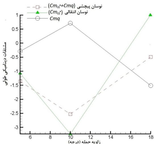
شکل 8 تغییرات مشتقات دینامیکی طولی با زاویه حمله متوسط، k=0/06 ، \bar{\alpha}=5^\circ ، V=30\text{m/s}
