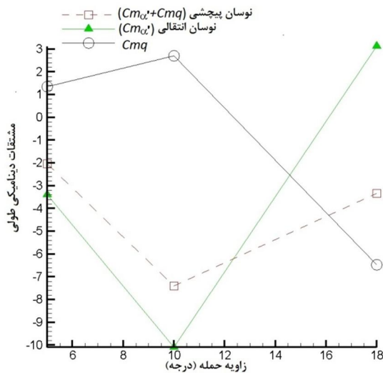
شکل 12 تغییرات مشتقات دینامیکی طولی با زاویه حمله متوسط، k=0/03, \bar{\alpha}=2^\circ V=60\text{m/s}
