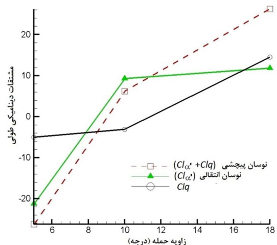
شکل 17 تغییرات مشتقات دینامیکی ضریب برآ با زاویه حمله متوسط، \bar{\alpha}=5^\circ ، V=30\text{m/s} ، k=0/06
