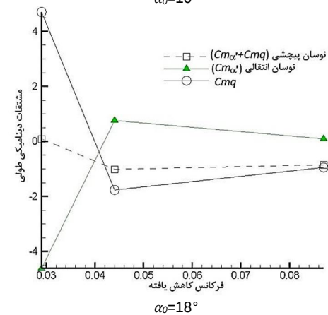
شکل 13 تغییرات مشتقات دینامیکی طولی با فرکانس کاهش یافته، V=30\text{m/s}
