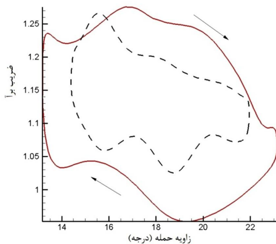
شکل 16 تغییرات ضریب برآ، \alpha_0=18^\circ ، \bar{\alpha}=5^\circ ، k=0/06 ، V=30\text{m/s}
