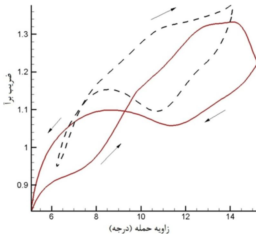
شکل 15 تغییرات ضریب برآ، \alpha_0=10^\circ ، \bar{\alpha}=5^\circ ، k=0/06 ، V=30\text{m/s}
