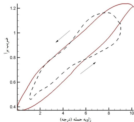
شکل 14 تغییرات ضریب برآ، \alpha_0=5^\circ ، \bar{\alpha}=5^\circ ، k=0/06 ، V=30\text{m/s}
