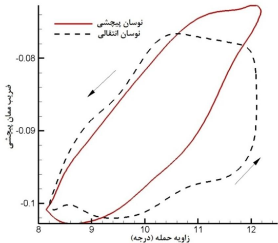
شکل 10 تغییرات ضریب ممان پیچشی، V=60\text{m/s}, k=0/03, \bar{\alpha}=2^\circ, \alpha_0=10^\circ
