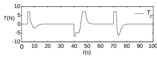
شکل 10 تعقیب فرمان هدایت و فرمان کنترل کانال سمت
