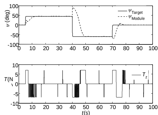
شکل 15 تعقیب فرمان هدایت و فرمان کنترل کانال سمت با ناهمراستایی تراستر و نویز اندازه‌گیری
