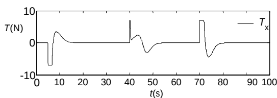
شکل 9 تعقیب فرمان هدایت و فرمان کنترل کانال فراز در زاویه 90 درج
