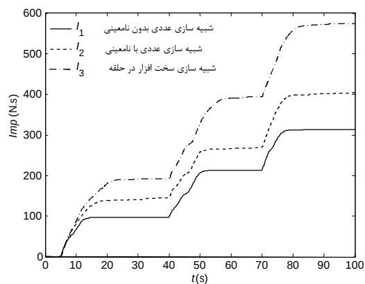
شکل 23 مجموع ضربه کنترل در مانور نمونه
