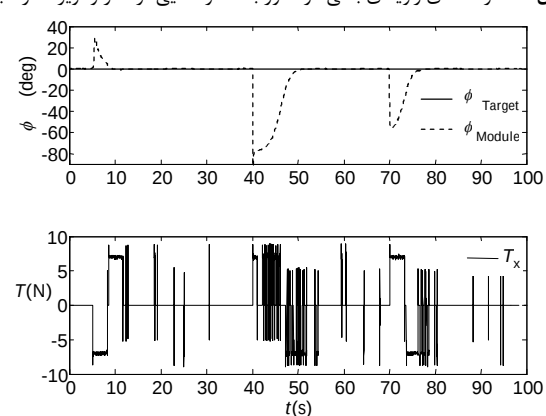
شکل 18 تعقیب فرمان هدایت و فرمان کنترل کانال چرخ با ناهمراستایی تراستر و نویز اندازه‌گیری در تست HIL
