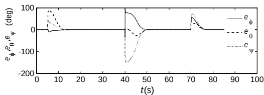
شکل 11 همگرایی بردار کوتاه‌ترین خط و زوایای اولیه
