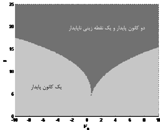
شکل ۳ تعداد و گونه‌ی اکسترممهای تابع چگالی احتمالی
