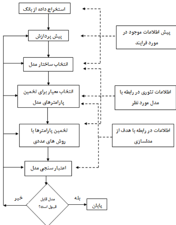
شکل ۲ فلوچارت طراحی سنسور نرم داده پایه
