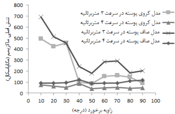
شکل ۶ توزیع تنش اصلی ماکزیمم در پوسته ها بر حسب زاویه برخورد
