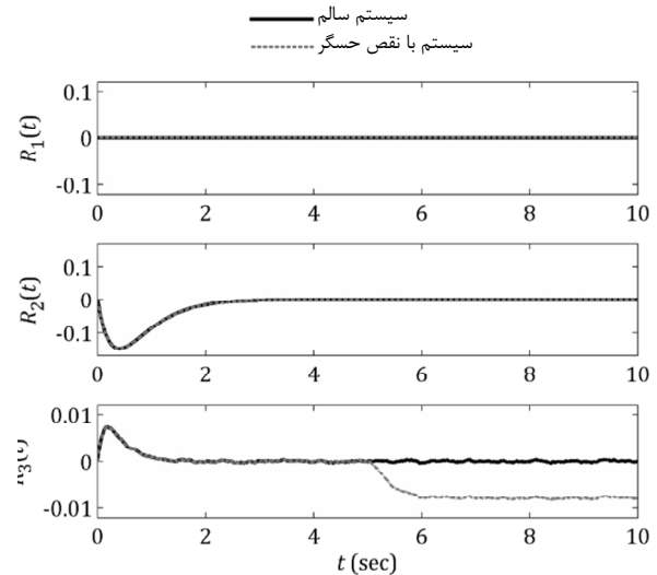
شکل ۱ مؤلفه‌های بردار مانده ایجاد شده توسط الگوریتم پیشنهادی این مقاله
