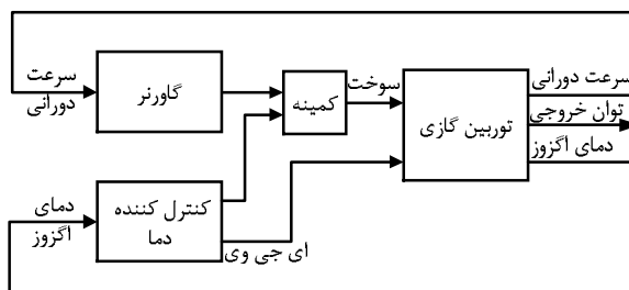
شکل ۲ دایگرام کنترلی توربین گازی در حالت جزیره‌ای
