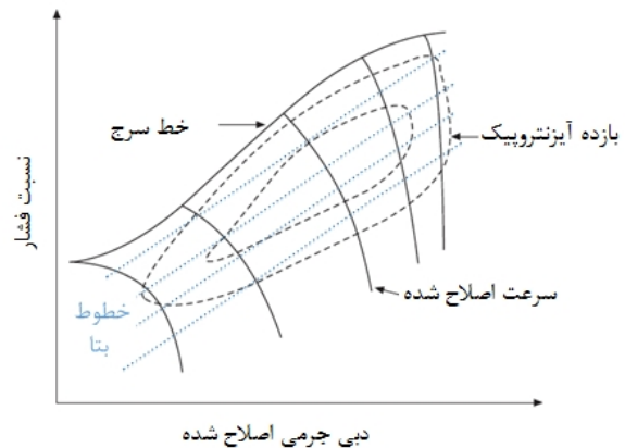
شکل ۴ شماتیک نگاشت کمپرسور
