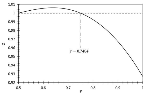
شکل 8 تغییرات \phi بر حسب \bar{r} برای n = 1.1 < n_{cr} و \Omega_{e1} = 1.3854
