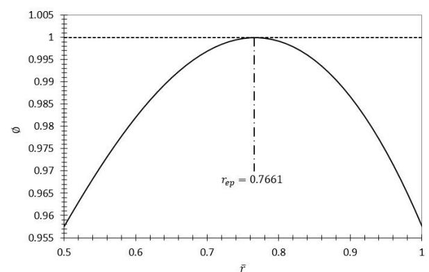
شکل 5 تغییرات \phi بر حسب \bar{r} را برای n = n_{cr} و \Omega = 1.39308 < \Omega_{cr}
