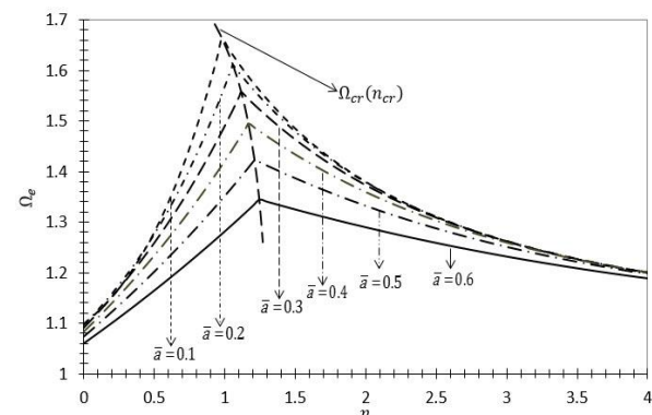
شکل 11 تغییرات سرعت حد دورانی بی‌بعد \Omega_\phi بر حسب n برای مقادیر مختلف شعاع داخلی بی‌بعد
