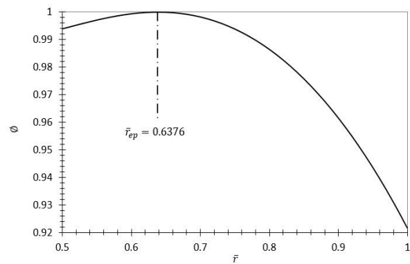
شکل 9 تغییرات \phi بر حسب شعاع بی بعد \bar{r} برای n = 1.1 < n_{cr} و \Omega = 1.3812 < \Omega_{cr}
