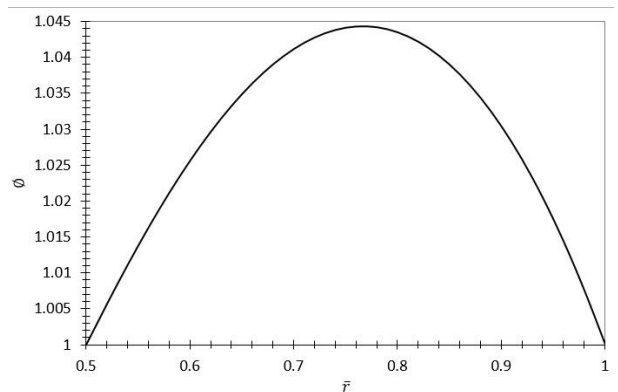
شکل 4 تغییرات متغیر \phi بر حسب شعاع بی بعد \bar{r} برای n_{cr} = 1.2109 و \Omega_{cr} = 1.4236
