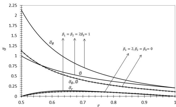
شکل 14 تاثیر تغییرات چگالی در طول شعاع دیسک
