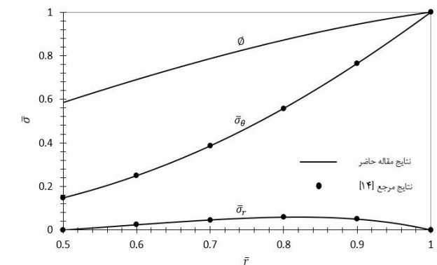
شکل 10 تغییرات تنش محیطی \bar{\sigma}_\theta ، تنش شعاعی \bar{\sigma}_r و \phi بر حسب \bar{r} برای n_{cr} > 2 و \Omega_{e2} = 1.33217 و مقایسه با نتایج مرجع [14]
