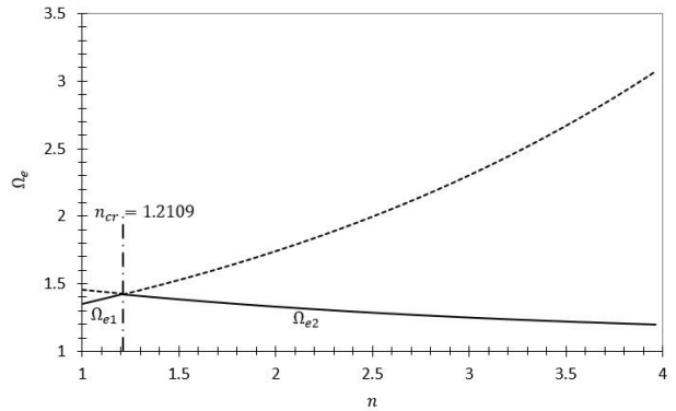
شکل 3 تغییرات سرعت حد بحرانی بی بعد \Omega_e بر حسب n برای \bar{a} = 0.5 و ثابتهای \beta_1 = \beta_2 = 2\beta_3 = 2
