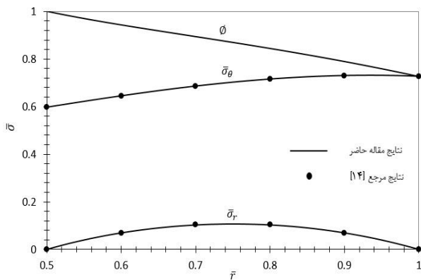
شکل 7 تغییرات تنش محیطی \bar{\sigma}_\theta ، تنش شعاعی \bar{\sigma}_r و \phi بر حسب \bar{r} برای n = 0.7424 < n_{cr} و \Omega_{e1} = 1.27165 و مقایسه با نتایج مرجع [14]
