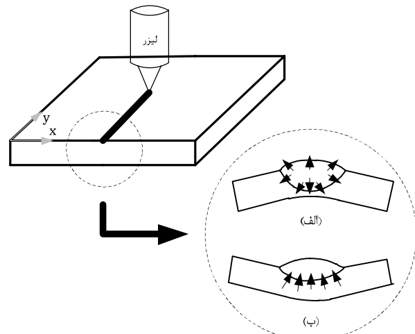
شکل 2 شماییک مکانیزم گرادیان دمایی (الف) خم منفی؛ (ب) خم دائمی ورق
