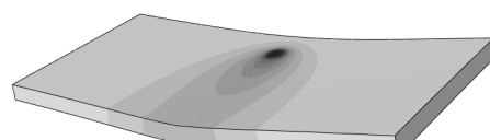
شکل 6 تصویر توزیع دمای ورق در حین فرآیند (الف) 0/36 ثانیه؛ (ب) 1/44 ثانیه؛ (پ) 2/52 ثانیه؛ (ت) 350 ثانیه
