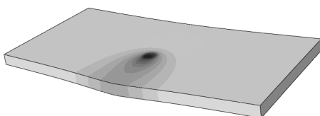
شکل 5 جابه‌جایی لبه‌ی آزاد ورق در حین فرآیند با مقیاس 1:15 (الف) 0/36 ثانیه؛ (ب) 1/44 ثانیه؛ (پ) 2/52 ثانیه؛ (ت) 350 ثانیه
