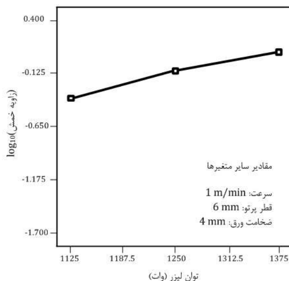
شکل 7 تأثیر توان بر زاویه خمش
