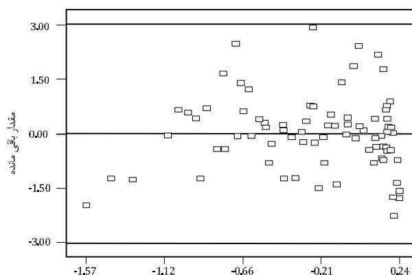
شکل 12 نمودار مقادیر باقی‌مانده در برابر مقادیر برازش یافته
