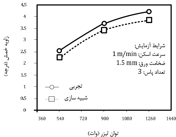
شکل 17 تغییر زاویه خمش برحسب تغییر توان لیزر
