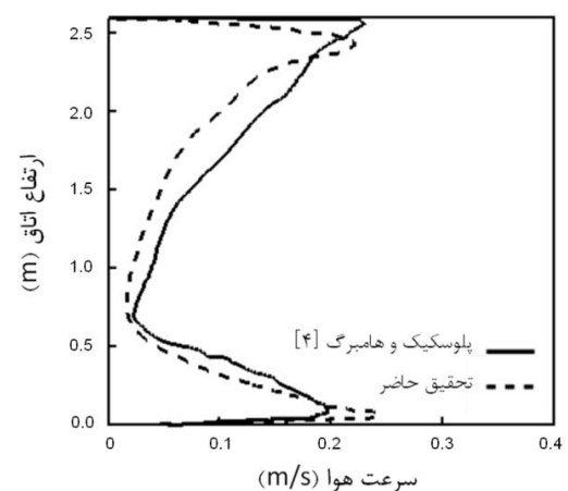
شکل 4 مقایسه نتایج تحقیق حاضر با نتایج پلوسیک و هامبرگ [4] به ازای تغییرات سرعت جریان هوا در مرکز اتاق با ارتفاع
