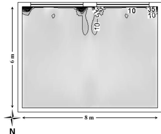
شکل 11 توزیع شاخص درصد نارضایتی حرارتی افراد (PPD) روی صفحه افقی به ارتفاع 0/6 متر در اتاقی دارای سیستم قرنیزی
