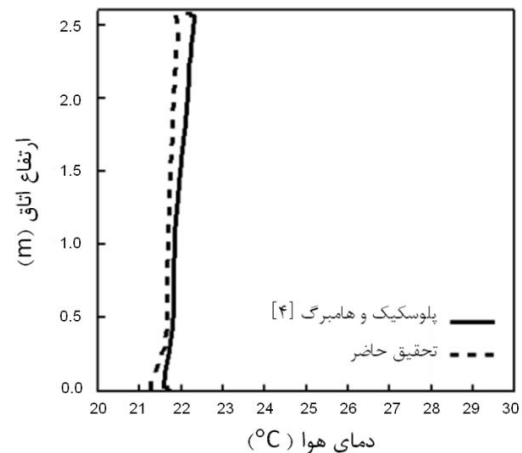
شکل 3 مقایسه نتایج تحقیق حاضر با نتایج پلوسیک و هامبرگ [4] به ازای تغییرات دمای هوا در مرکز اتاق با ارتفاع
