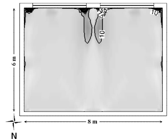
شکل 12 توزیع شاخص درصد نارضایتی حرارتی افراد (PPD) روی صفحه افقی به ارتفاع 1/1 متر در اتاقی دارای سیستم قرنیزی
