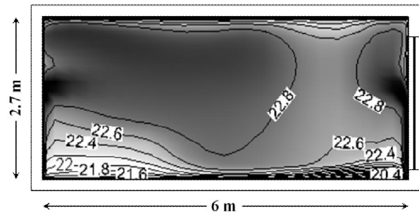
شکل 6 توزیع دمای هوا بر روی صفحه تقارن در اتاقی دارای سیستم قرنیزی با در نظر گرفتن اثرات نفوذ هوا از درز پنجره
