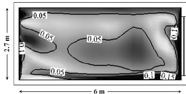
شکل 7 توزیع سرعت هوا بر روی صفحه تقارن در اتاقی دارای سیستم قرنیزی با در نظر گرفتن اثرات نفوذ هوا از درز پنجره
