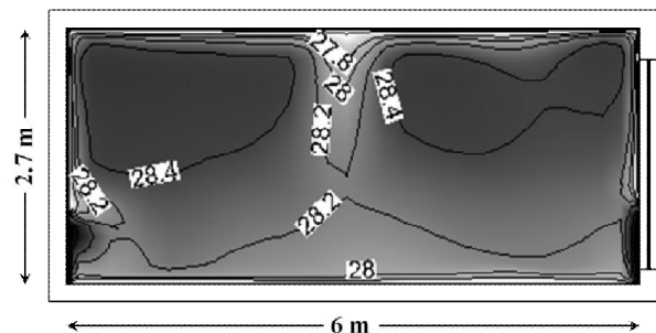
شکل 8 توزیع دمای هوا بر روی صفحه تقارن در اتاقی دارای سیستم قرنیزی بدون در نظر گرفتن اثرات نفوذ هوا از درز پنجره
