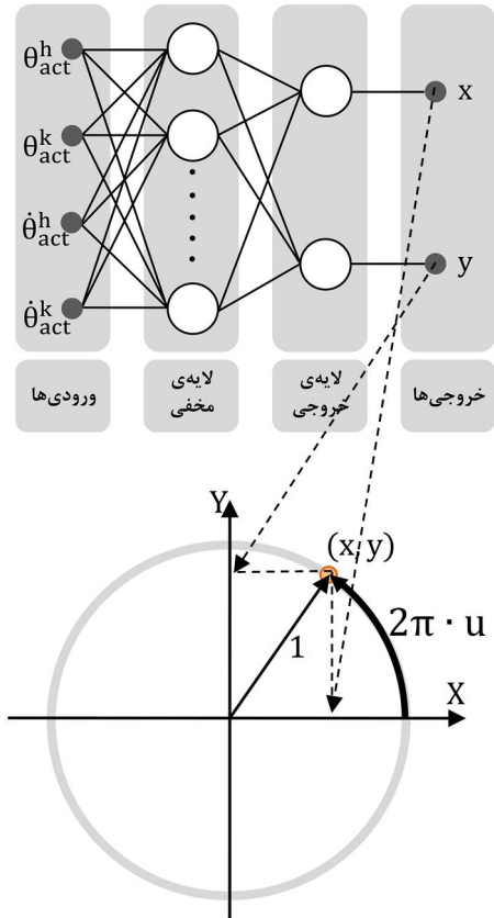
شکل 3 در الگوریتم تشخیص فاز حرکت، شبکه عصبی زوایای و سرعت زاویه‌ای واقعی مفاصل را دریافت می‌کند و فاز حرکت (مقدار u ) را تخمین می‌زند
