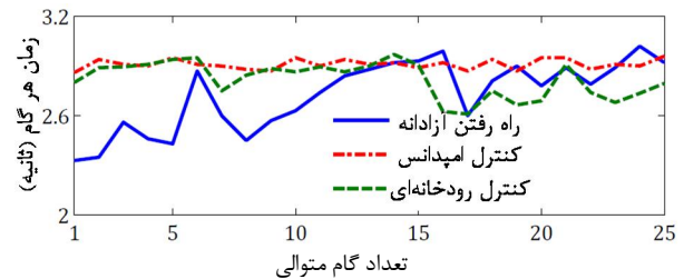
شکل 15 دوره‌ی زمانی گام بیمار در راه رفتن آزادانه، به کمک کنترل امپدانس و به کمک کنترلر رودخانه‌ای
