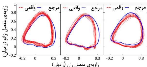
شکل 9 مسیر مرجع و مسیر واقعی مفصل زانو و ران (در فضای مفصل) برای سه فرد سالم در راه رفتن به کمک کنترل امپدانس
