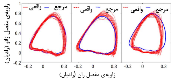
شکل 11 مسیر مرجع و مسیر واقعی مفاصل زانو و ران (در فضای مفاصل) برای سه فرد سالم در راه رفتن به کمک کنترلر رودخانه‌ای
