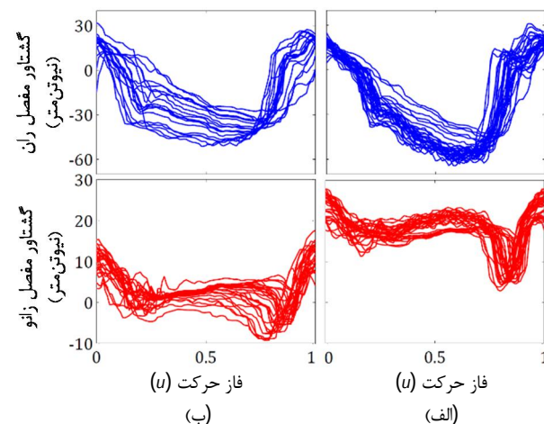
شکل 16 گشتاورهای اعمالی به مفاصل ران و زانو بیمار در دو حالت (الف) کنترل امپدانس و (ب) کنترل رودخانه‌ای
