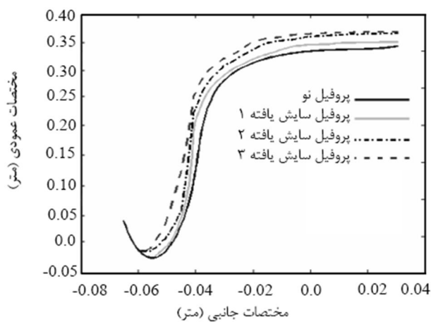
شکل 17 هندسه پروفیل‌های چرخ S1002 در چهار حالت نو، سایش یافته 1،
