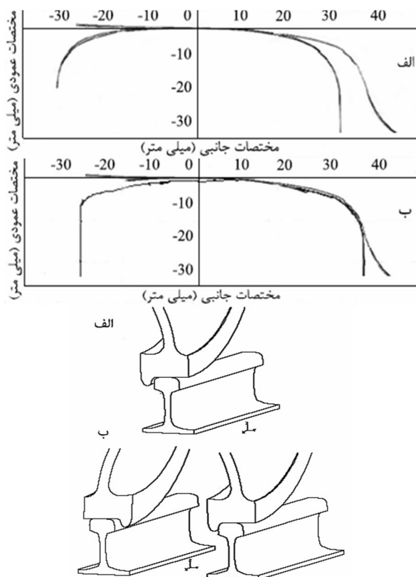
شکل 2 الف - حالت مسیر مستقیم (تماس لبه چرخ)، ب - حالت مسیر منحنی الخط
