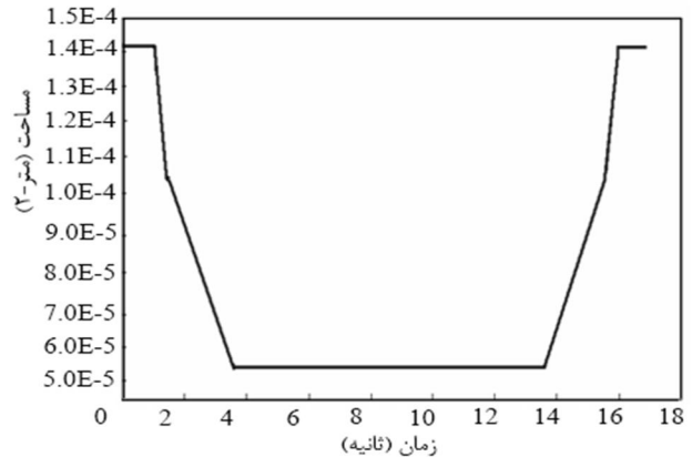
شکل 10 تغییرات مساحت بیضی تماسی هر ترز
