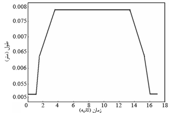
شکل 8 تغییرات نیم‌محور طولی بیضی تماسی هر ترز a
