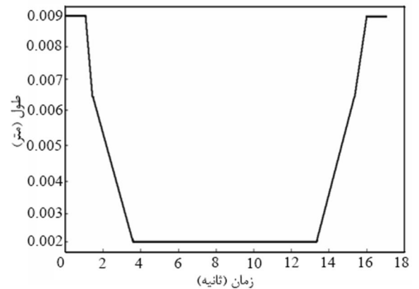
شکل 9 تغییرات نیم‌محور عرضی بیضی تماسی هر ترز b
