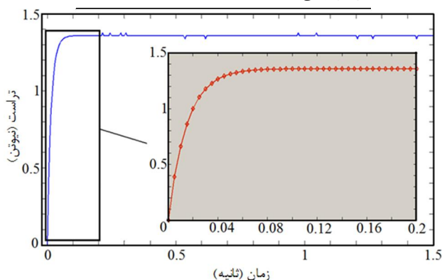
شکل 18 نتایج تست نهایی رانشگرها برای بررسی رانش و پاسخ زمانی سولونوید
