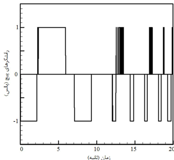
شکل 22 نمودار عملکرد رانشگرهای محور پیچ
