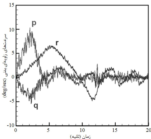
شکل 20 نمودار سرعت‌های زوایای شبیه‌ساز در راستای محورهای بدنی
