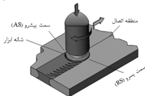
شکل 1 طرح‌واره فرایند جوشکاری اصطکاکی اغتشاشی [2]
