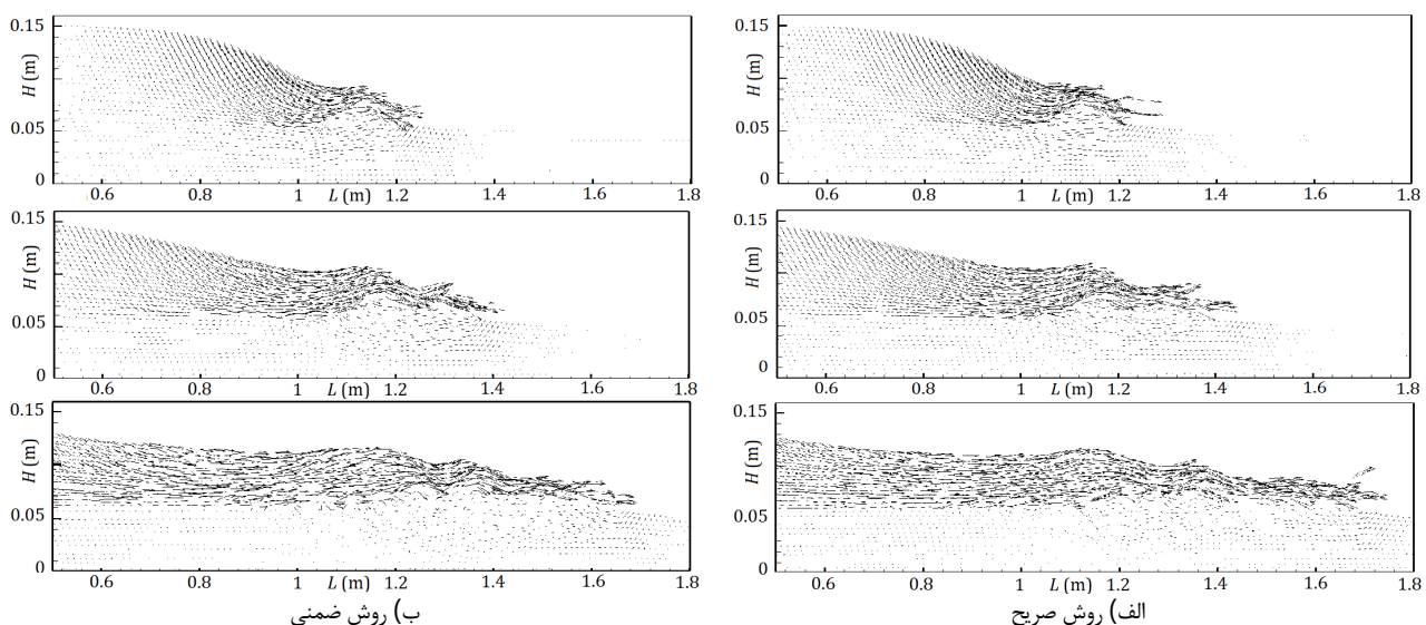
شکل 14 ارزیابی بردارهای سرعت روش های صریح و ضمنی در زمان های 0.05، 0.25 و 1 ثانیه (از بالا به پایین)
