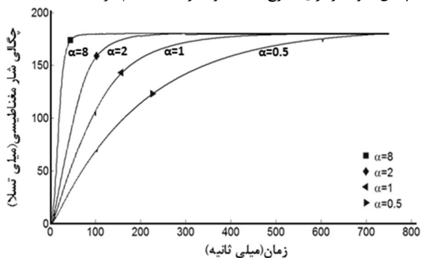
شکل 10 تغییرات چگالی شار مغناطیسی اعمالی به کویل
