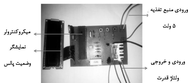
شکل 9 مجموعه طراحی شده برای اعمال جریان کنترل شده
