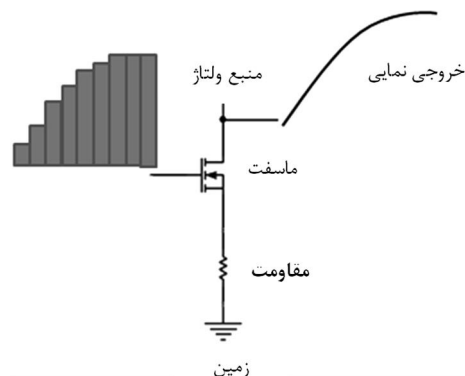
شکل 8 مدار الکتریکی
