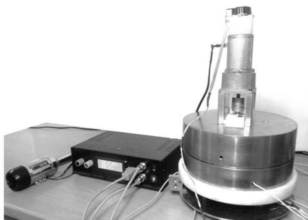
شکل 1- ب کوپلینگ آزمایشگاهی اندازه گیری تنش برشی
