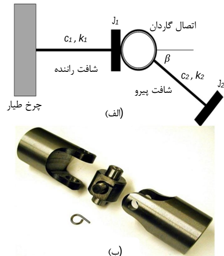
شکل 1 الف) شماتیک یک سیستم دوار ب) اجزای یک اتصال گاردان.
