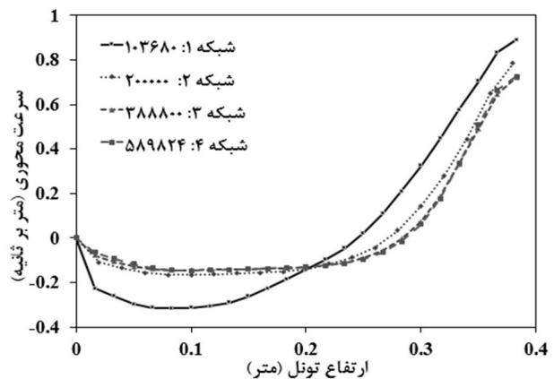
شکل 3 توزیع سرعت نسبت به ارتفاع در فاصله 2/7 متری از محل آتش‌سوزی در شبکه‌های مختلف محاسباتی برای نرخ گرمای آزاد شده 12/9 کیلووات
