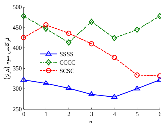
شکل 20 تاثیر شرایط مرزی مختلف روی فرکانس سوم صفحه ساندویچی (90_{6-n}/0_6/90_n)_s / MRE / (90_{6-n}/0_6/90_n)_s
