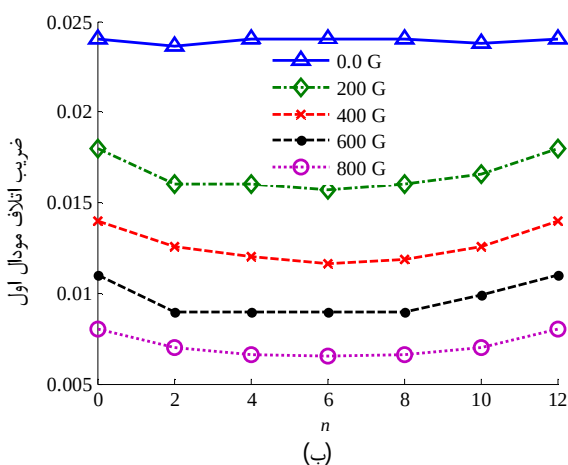
شکل 4 تاثیر تعداد لایه‌های صفر درجه و میدان مغناطیسی روی (الف) فرکانس اول و (ب) ضریب اتلاف مودال اول صفحه ساندویچی (90_{12-n}/O_n)_s / MRE / (90_{12-n}/O_n)_s
