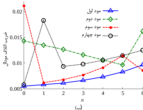
شکل 16 تاثیر فاصله لایه‌های صفر درجه تا صفحه میانی بر (الف) فرکانس‌ها (ب) ضریب اتلاف مودال صفحه ساندویچی با شرط مرزی SCSC
