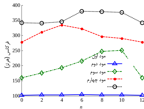
شکل 7 تاثیر تعداد لایه‌های صفر درجه بر فرکانس‌های صفحه ساندویچی SSSS با شرط مرزی SSSS
