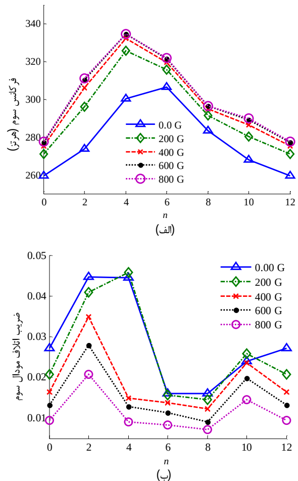
شکل 8 تاثیر تعداد لایه‌های صفر درجه و میدان مغناطیسی روی (الف) فرکانس سوم و (ب) ضریب اتلاف مودال سوم صفحه ساندویچی
