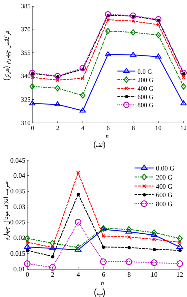
شکل 6 تاثیر تعداد لایه‌های صفر درجه و میدان مغناطیسی روی (الف) فرکانس چهارم و (ب) ضریب اتلاف مودال سوم صفحه ساندویچی
