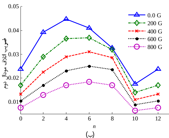
شکل 5 تاثیر تعداد لایه‌های صفر درجه و میدان مغناطیسی روی (الف) فرکانس دوم و (ب) ضریب اتلاف مودال دوم صفحه ساندویچی (90_{12-n}/O_n)_s / MRE / (90_{12-n}/O_n)_s
