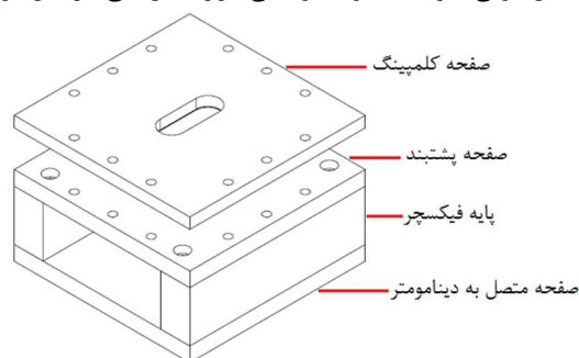
شکل 10 اجزای فیکسچر فرایند شکل‌دهی تدریجی
