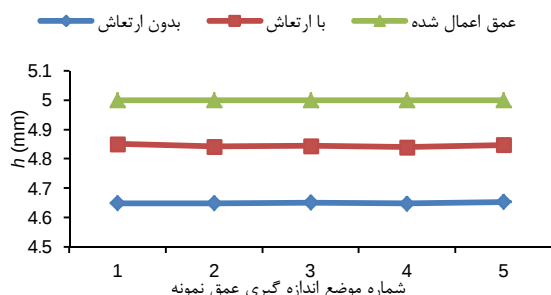
شکل 19 نمودار مقایسه‌ی عمق نمونه‌های شکل‌دهی شده
