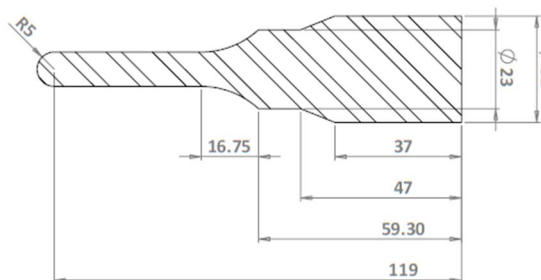
شکل 5 طراحی ابزار سرنیمکروی مرتعش به قطر 10 میلی‌متر
