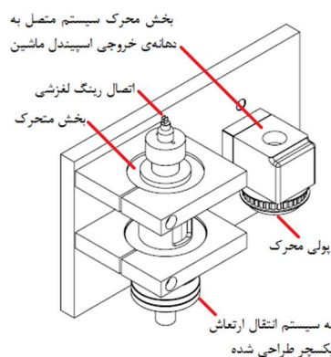
شکل 2 طراحی فیکسچر
