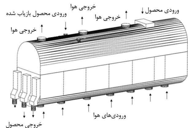
شکل 1 نمای خشک کن مورد مطالعه
