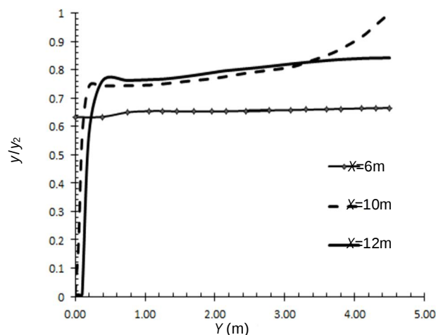
شکل 11 نمودار توزیع ارتفاعی رطوبت در فاز جامد
