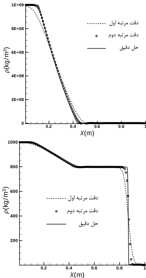
شکل 3 لوله ضربه گاز-مایع، مقایسه نتایج عددی (سمبل) با نتایج دقیق (خط پر) [10]. تعداد مش 1000 و CFL = 0/8
