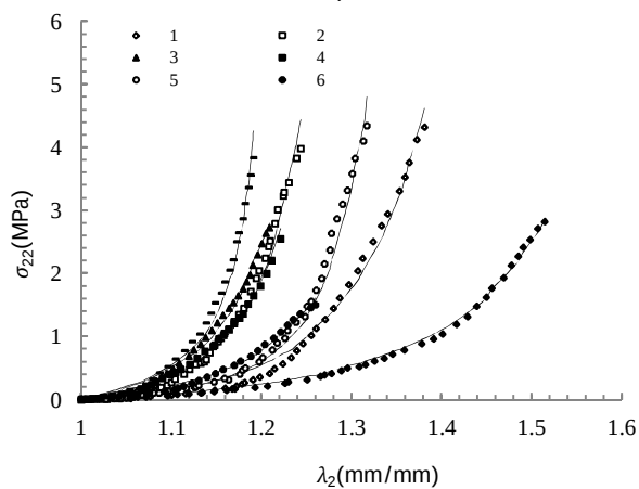
شکل 5 مقایسه نمودارهای تنش-کشش حاصل از مدل فانگ با داده های تجربی در (الف) راستای پیرامونی و (ب) راستای طولی
