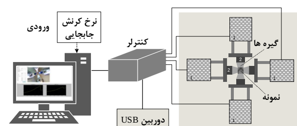
شکل 1 شماتیک از دستگاه کشش دوجوری (1. میکروموتورها، 2. لودسل ها)
