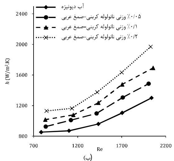
شکل 8 ضریب انتقال حرارت جابجایی محلی بر اساس عدد رینولدز در غلظت‌های وزنی مختلف، الف) x/D=14/3 و ب) x/D=128/57
