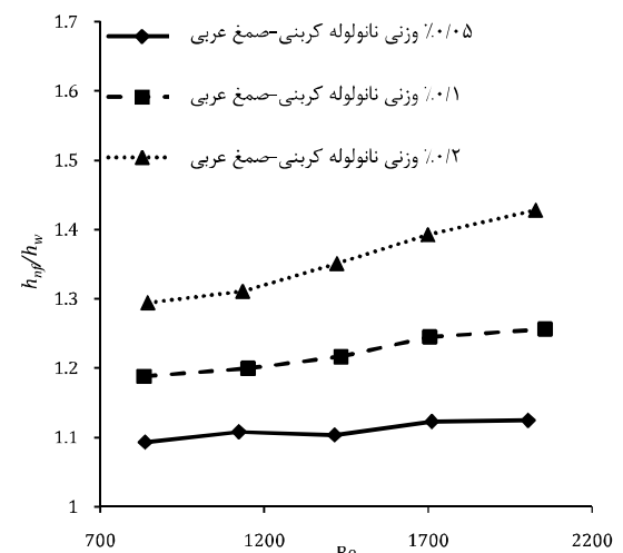
شکل 9 نسبت ضریب انتقال حرارت جابجایی متوسط نانوسیال به آب دیونیزه بر حسب عدد رینولدز متوسط در غلظت‌های وزنی مختلف
