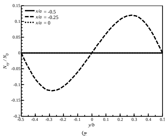
شکل 5 تغییرات منته‌های نیروی داخل صفحه‌ای در سه موقعیت مختلف برای بارگذاری کسینوسی الف) منته‌های نیروی N_x ، ب) منته‌های نیروی N_y ، ج) منته‌های نیروی N_{xy} .
