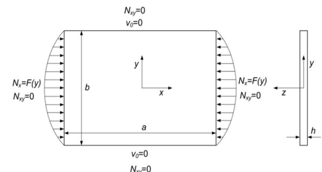
شکل 1 ورق مستطیلی با بارگذاری غیریکنواخت در لبه‌ها
