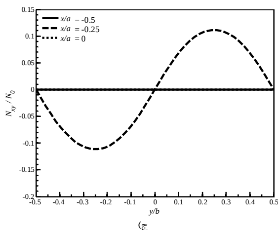
شکل 6 تغییرات منته‌های نیروی داخل صفحه‌ای در سه موقعیت مختلف برای بارگذاری مثلثی الف) منته‌های نیروی N_x ، ب) منته‌های نیروی N_y ، ج) منته‌های نیروی N_{xy} .
