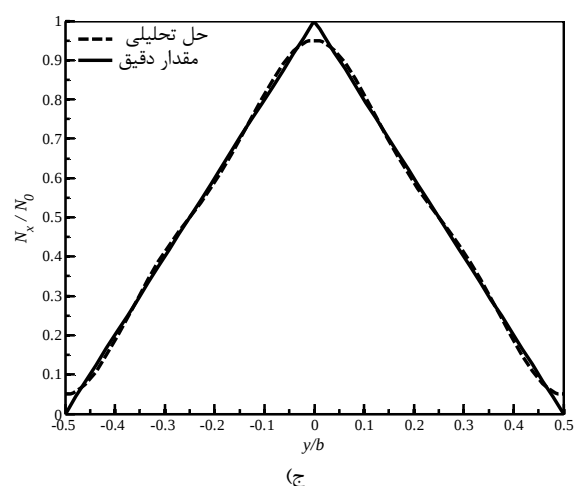
شکل 3 مقایسه مقدار به‌دست آمده از حل تحلیلی برای N_x در لبه سمت راست و چپ ورق با مقدار دقیق آن، (الف) بارگذاری سهمی (شکل، ب) بارگذاری کسینوسی و ج) بارگذاری مثلثی.
