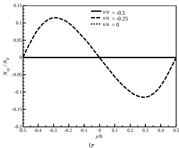
شکل 4 تغییرات منته نیروی‌های داخل صفحه‌ای در سه موقعیت مختلف برای بارگذاری سهمی (شکل الف) منته نیروی N_x ، (ب) منته نیروی N_y ، (ج) منته نیروی N_{xy} .
