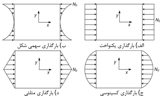
شکل 2 حالت‌های مختلف بارگذاری غیریکنواخت یک ورق مستطیلی.
