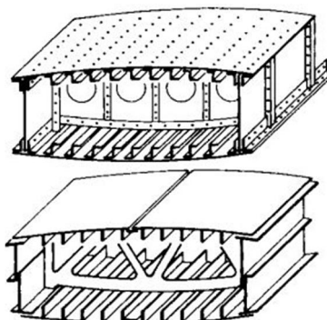
شکل 2، بنا بر تقویت شده در دو حالت تقویت کننده یکبارجه و برچ شده [12]
