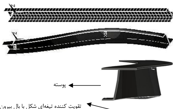
شکل 9 شکل مود کمانش اول پل تقویت شده یکپارچه با تقویت کننده تیغه‌ای با بال بیرون زده در یک گام
