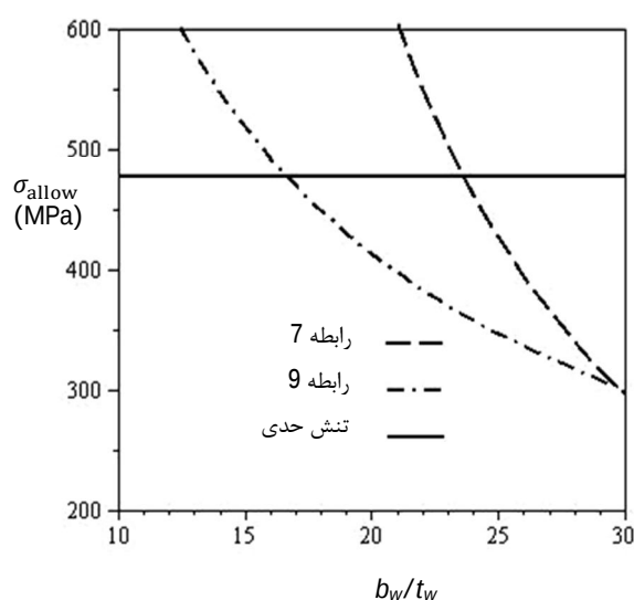
شکل 5 مقایسه روابط 7 و 9 برای پیش‌بینی کریپلینگ استرینگر
