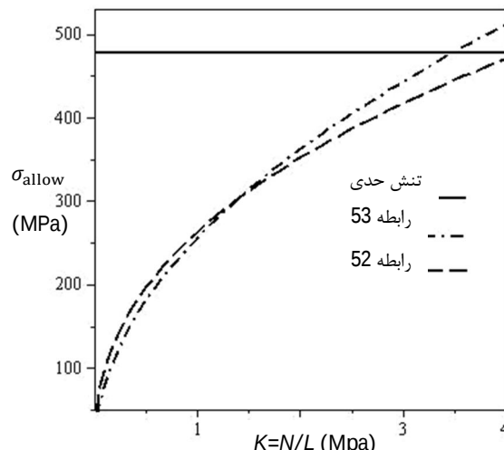
شکل 7 مقایسه مقدار تنش به‌شینه از دو روش مختلف بر اساس شناسه سازه
