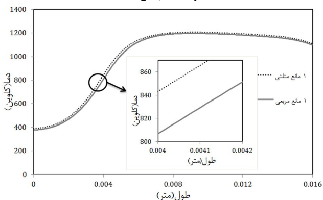
شکل 13 پروفیل توزیع دمای خط جریان برای احتراق هیدروژن-هوا با سرعت
