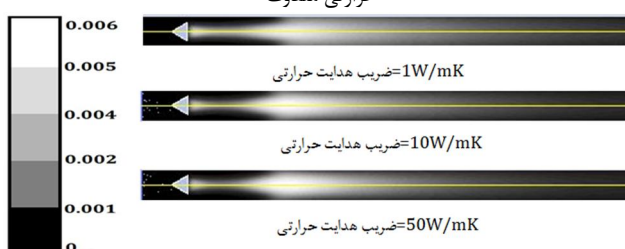
شکل 24 کانتور کسر جرمی رادیکال OH برای احتراق هیدروژن-هوا با سرعت ثابت ورودی 10 m/s و نسبت هم‌ارزی ثابت 0/5 و به ازای ضریب هدایت حرارتی‌های مختلف
