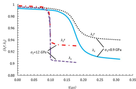
شکل 7 تاریخچه زمانی کشیدگی پلاستیک و کشیدگی کل برای 8/9 و 12 GPa.
