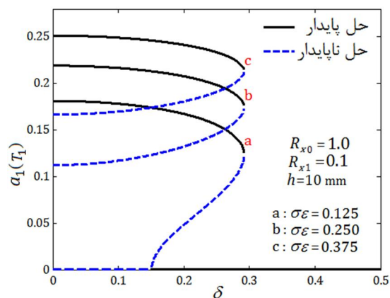
شکل 11 تغییرات دامنه تشدید با پارامتر میرایی، در غیاب بستر الاستیک
