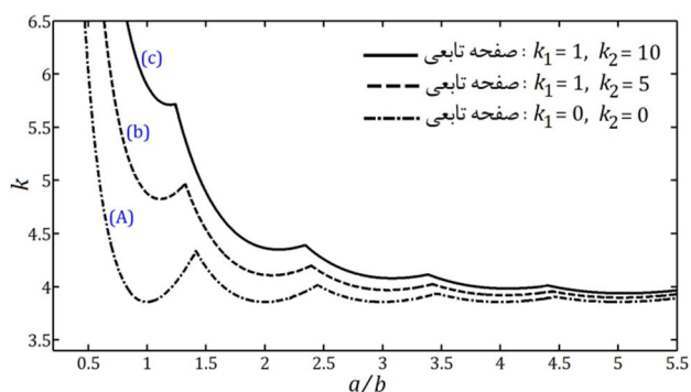
شکل 2- ب تغییرات ضریب کماتش صفحه تابعی با شرایط مرزی تکیه‌گاهی ساده متحرک در برابر پارامتر نسبت ابعاد (a/b) با وجود بستر الاستیک در سه حالت از مقادیر ضرایب سفتی بستر، A)
