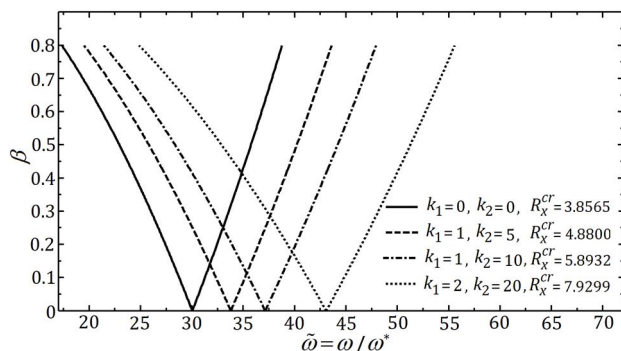
شکل 4-الف تقریب مرتبه اول ناحیه اصلی ناپایداری دینامیکی صفحه تحت نیروی درون-صفحه‌ای تک محوره ( \alpha=0.4 ) برای چهار حالت از ضرایب بستر.
