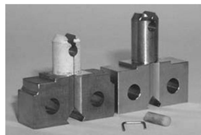
شکل 10 نمونه فیکسچر واقعی [25]
