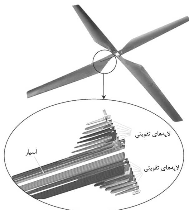
شکل 1 نمای انفجاری پره روتور یک بالگرد
