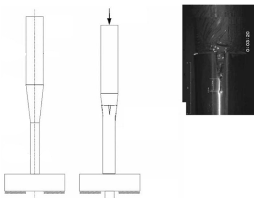
شکل 17 روش آزمایش قالب مخروطی داخلی [28]
