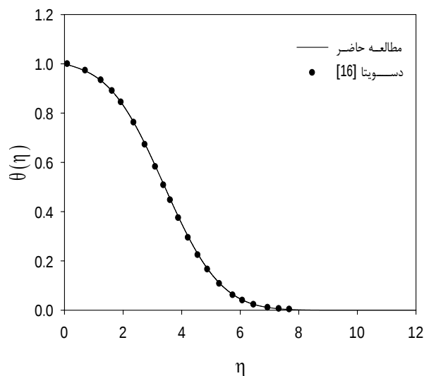
شکل 2 پروفیل دما در سیال خالص به ازای n=0.01 ، \lambda=-0.03 و Pr=0.7
