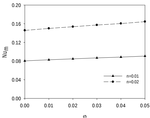
شکل 11 تغییرات پارامتر معرف عدد نوسلت Num نسبت به \phi در n=0.01, 0.02 به ازای \lambda = 0.04
