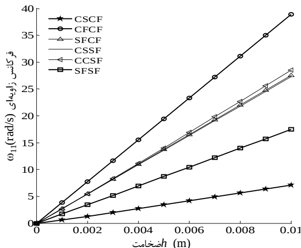
شکل 5 تغییرات فرکانس طبیعی بر حسب ضخامت ورق با نسبت ابعادی C = 0/1 و \frac{b}{a} = \frac{2}{3} ترک به طول نسبی
