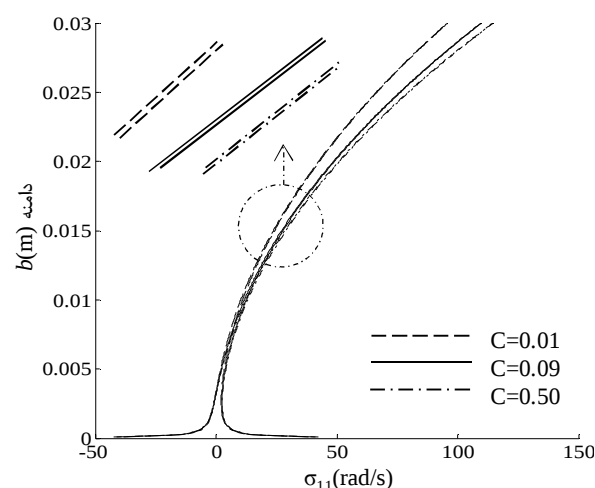
شکل 10 منحنی پاسخ فرکانسی ورق CCSCF با ابعاد 3 \times 2 \times 0/01m و مقادیر مختلف طول نسبی ترک 2C
