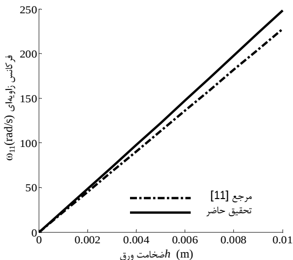
شکل 2 تغییرات فرکانس طبیعی بر حسب ضخامت برای ورق CCFF با ابعاد 1 \times 1 m و 0/5 و ترک به طول 2c = 0/1 m
