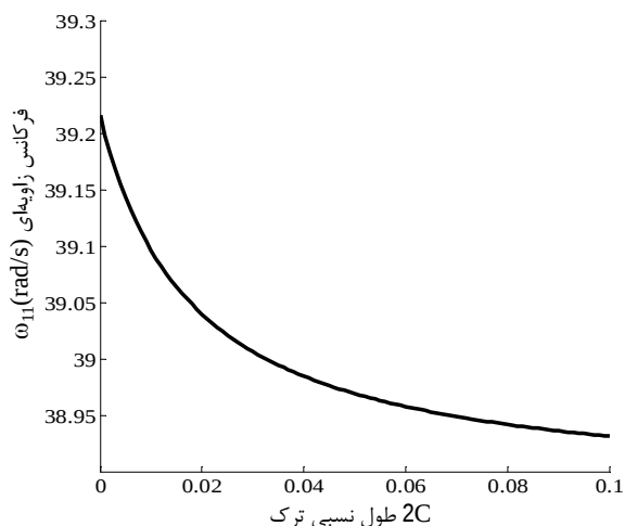
شکل 6 تغییرات فرکانس طبیعی بر حسب طول نسبی ترک برای ورق CFCF با نسبت ابعادی \frac{b}{a} = \frac{2}{3} و ضخامت h = 0/01m
