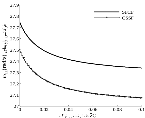
شکل 7 تغییرات فرکانس طبیعی بر حسب طول نسبی ترک برای ورق با نسبت ابعادی \frac{b}{a} = \frac{2}{3} و ضخامت h = 0/01m
