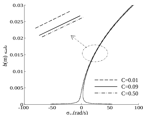
شکل 9 منحنی پاسخ فرکانسی ورق SFCF با ابعاد 3 \times 2 \times 0/01m و مقادیر مختلف طول نسبی ترک 2C
