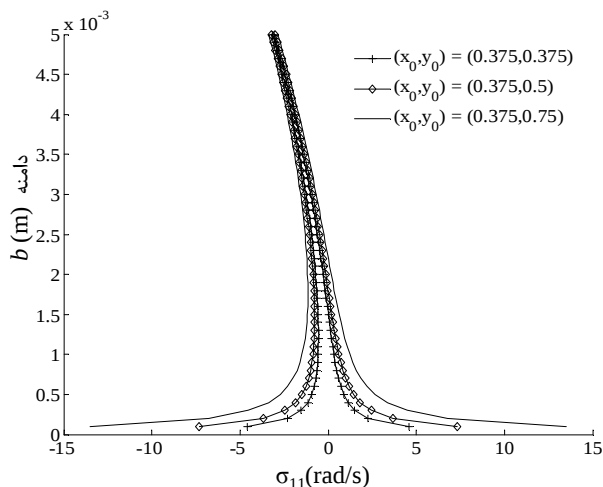
شکل 4 منحنی پاسخ فرکانسی ورق CCFF با ابعاد 1 \times 1 \times 0/01m و به ازای نقاط مختلف اعمال بار متمرکز 10 N
