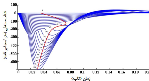
شکل 10 پیش‌بینی مدل از شتاب خودرو در سرعت‌های بین 0 تا 100 کیلومتر در ساعت
