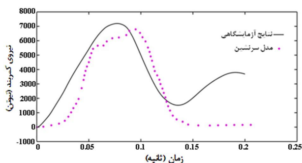
شکل 16 مقایسه نیروی وارد به سینه در مدل چندین عضوی و نتایج آزمایشگاهی
