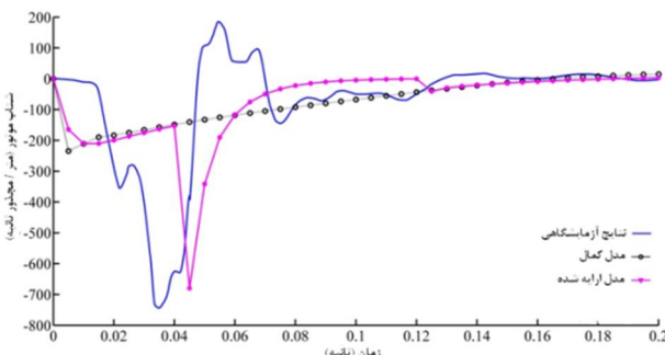
شکل 5 مقایسه شتاب موتور دو مدل با نتیجه آزمایش در سرعت 48 کیلومتر بر ساعت [17]
