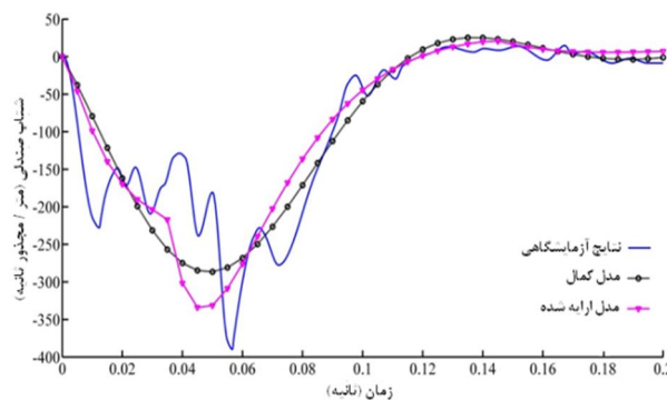
شکل 6 مقایسه شتاب صندلی دو مدل با نتیجه آزمایش در سرعت 56 کیلومتر بر ساعت [17]
