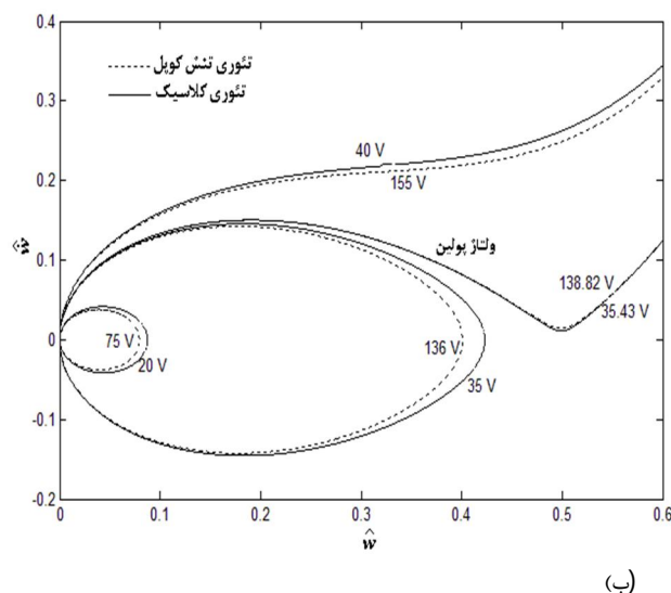
شکل 8 صفحه فازی به ازاء ولتاژهای پله متفاوت (الف. میکروتیر طلا و ب. میکروتیر نیکل)
