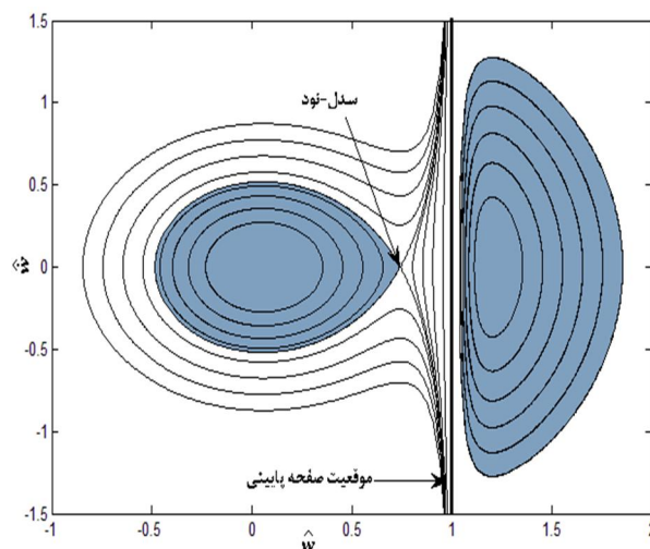
شکل 4 صفحه فازی برای میکروتیر طلا به ازاا شرایط اولیه مختلف
