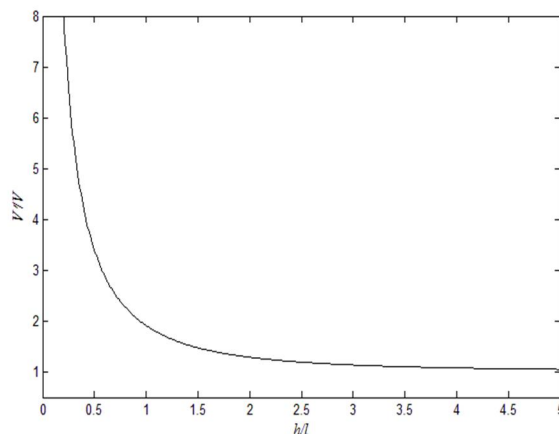
شکل 5 تغییرات نسبت ولتاژ پولین بر حسب h/l
