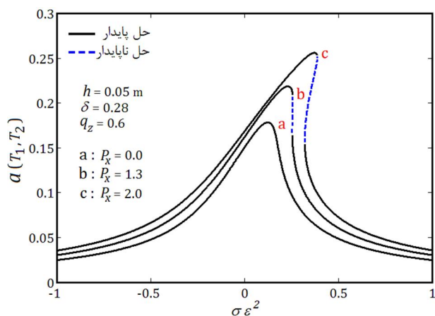
شکل 11 منحنی های مشخصه پاسخ فرکانسی برای سه مقدار از دامنه نیروی تحریک درون - صفحه ای P_x = 0 ، P_x = 1.3 و P_x = 2
