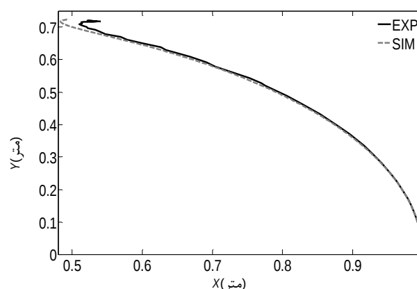
شکل 11 مسیرهای بار ماکزیمم در صفحه XY
