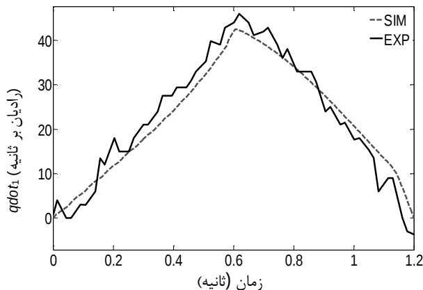
شکل 7 سرعت زاویه‌ای مفصل اول برای مسیرهای بار ماکزیمم
