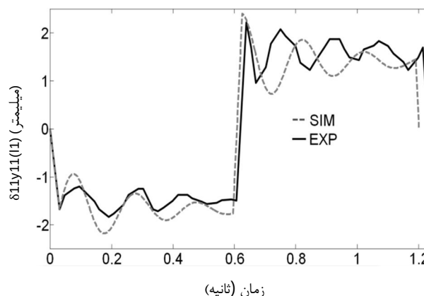
شکل 9 خیز نقطه انتهایی عضو اول نسبت به زمان
