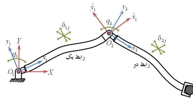
شکل 1 شماتیک ربات دو عضوی انعطاف‌پذیر
