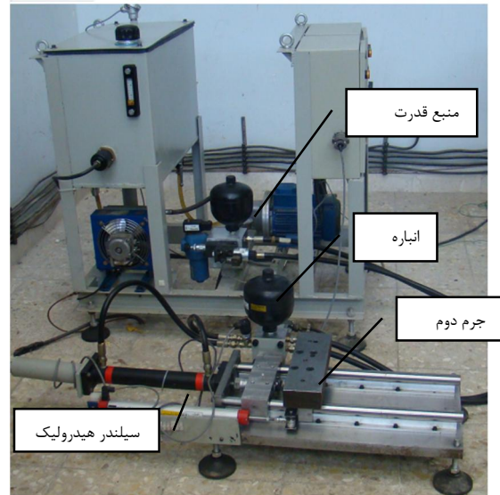
شکل 10 میز سرویهیدرولیک
