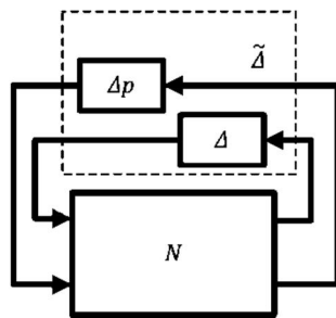
شکل 9 تبدیل بلوک دیاگرام به M-D
