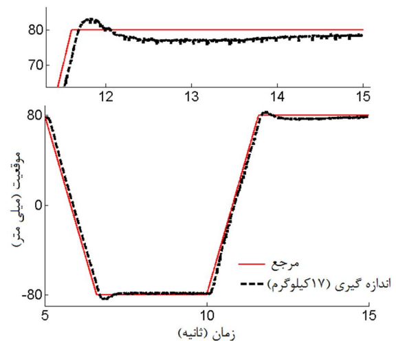
شکل 20 نتایج پیاده‌سازی کنترلگر مقاوم دو درجه آزادی
