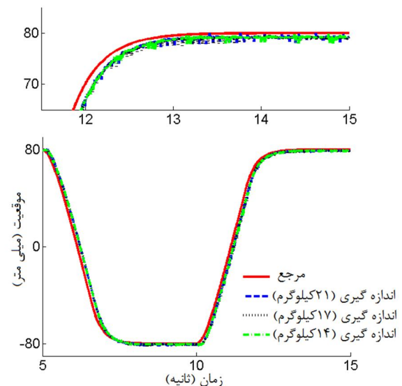
شکل 21 نتایج پیاده‌سازی کنترلگر مقاوم دو درجه آزادی
