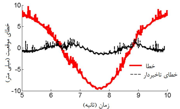
شکل 19 نمودار زمانی خطای اندازه‌گیری شده
