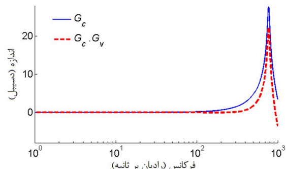
شکل 12 نمودار پاسخ فرکانسی تابع دینامیکی شیرسرو و سیلندر هیدرولیک
