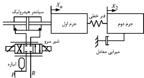
شکل 11 مدل میز سرویهیدرولیک
