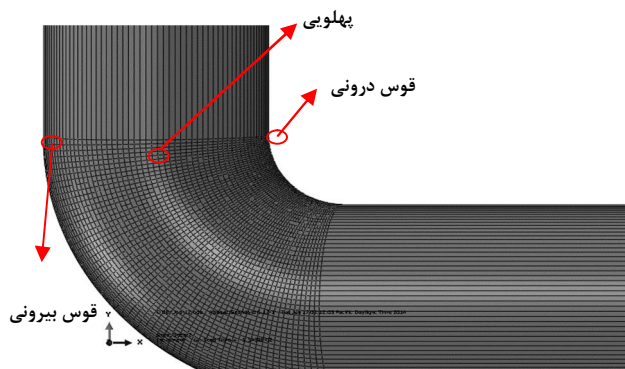
شکل 5 مدل اجزای محدود از لوله زانویی تحت فشار ثابت و خمش سیکلی
