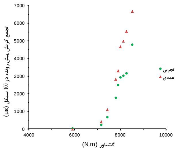
شکل 13 کرنش های پیش رونده به دست آمده از نتایج تجربی و عددی برای نمونه CSXO
