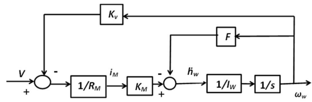
شکل 2 مدل پایه یک طرح تغییر ممتموم مثلاً چرخ عکس‌العملی
