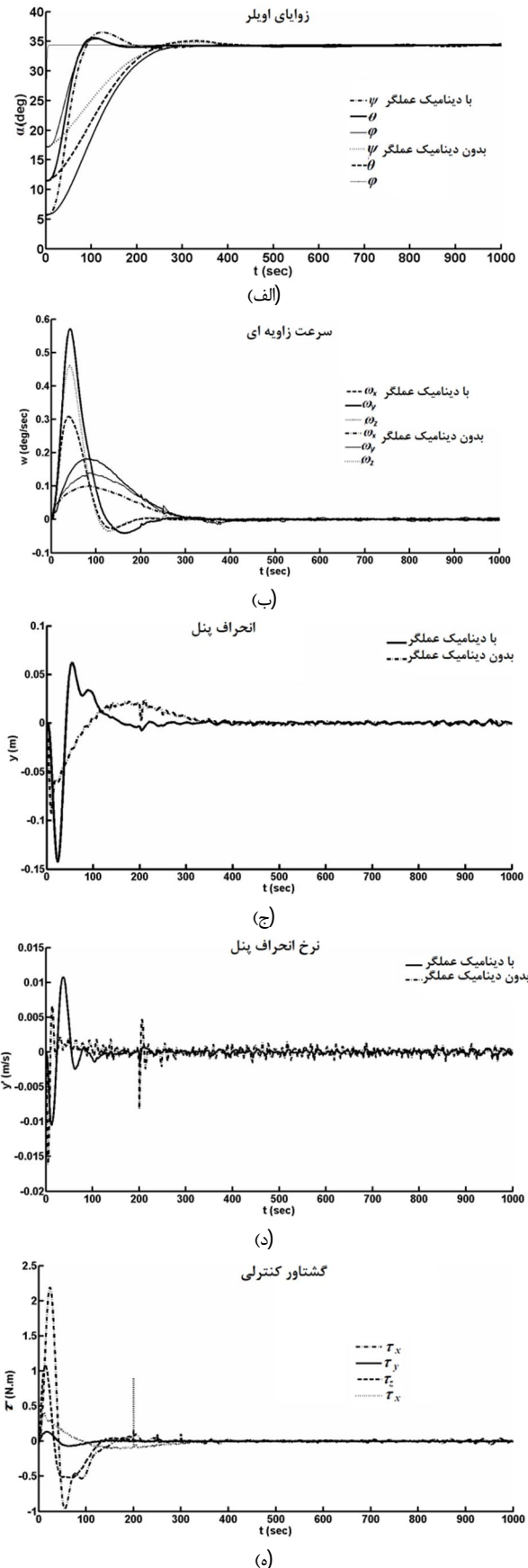
شکل 6 الف) زوایای اوایلر ب) سرعت زاویه‌ای ج) انحراف بالک د) نرخ انحراف بالک ه) گشتاور کنترلی، ماهواره الاستیک فضایی، روش کنترلی ترکیبی، مقایسه پاسخ‌ها با دینامیک عملگر و بدون آن
