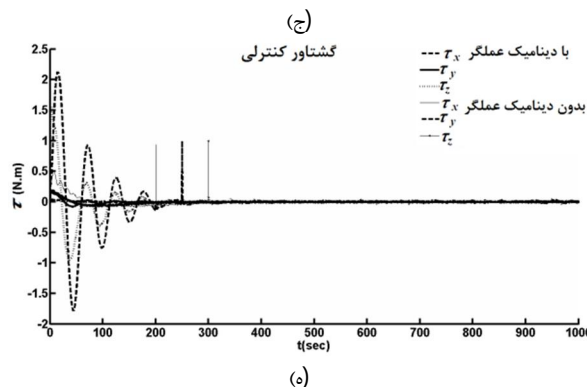
شکل 5 الف) زوایای اوایلر ب) سرعت زوایه‌ای ج) انحراف پیل د) نرخ انحراف پیل ه) گشتاور کنترلی، روش کنترلی وارون دینامیک، مقایسه پاسخ‌ها با در نظر گرفتن دینامیک عملگر و بدون آن
