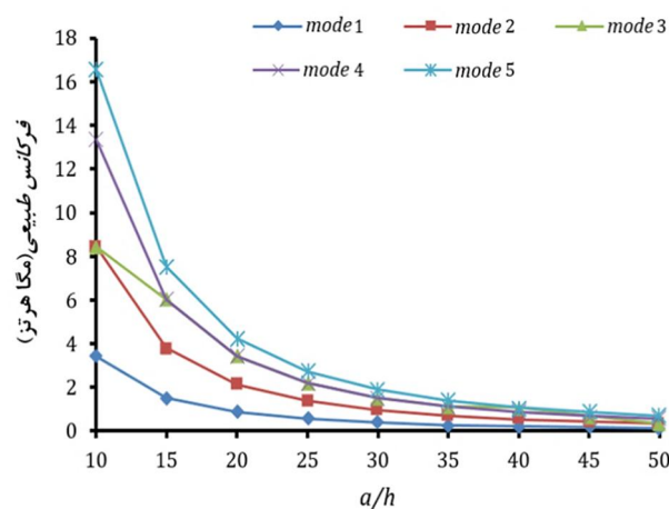
شکل 8 نمودار تغییرات پنج فرکانس اول نانورق تابعی مدرج بر حسب تغییرات نسبت طول به ضخامت ورق
