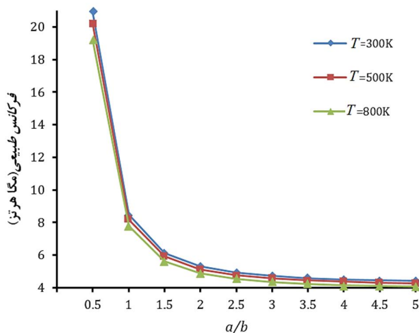
شکل 10 نمودار تغییرات فرکانس پایه نانورق تابعی مدرج بر حسب تغییرات نسبت ضخامت به پارامتر مقیاس طول برای دماهای محیطی مختلف
