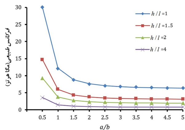
شکل 9 نمودار تغییرات فرکانس پایه نانورق تابعی مدرج بر حسب تغییرات نسبت طول به عرض ورق برای نسبت ضخامت به پارامتر مقیاس طول مختلف
