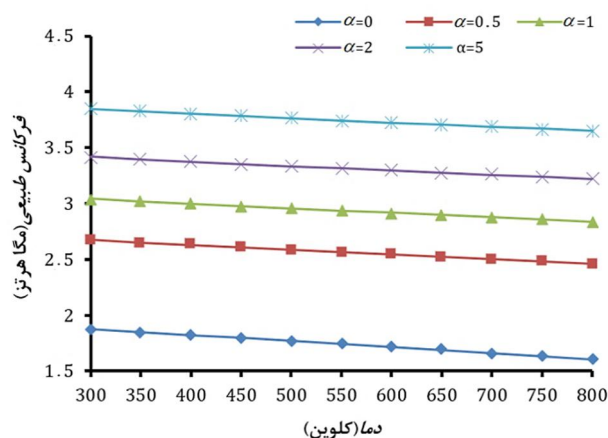
شکل 7 نمودار تغییرات فرکانس پایه نانورق تابعی مدرج بر حسب تغییرات دمای محیطی برای ضرایب نسبت حجمی توانی مختلف
