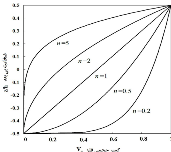
شکل 2 تغییرات کسر حجمی فلز بر حسب ضخامت بی بعد برای ضرایب نسبت حجمی توانی مختلف
