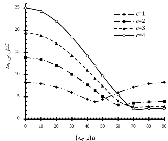
شکل 14 بررسی تغییرات تنش بی‌بعد برای چیدمان [0/90]_s بر حسب زاویه اعمال بار در C های مختلف
