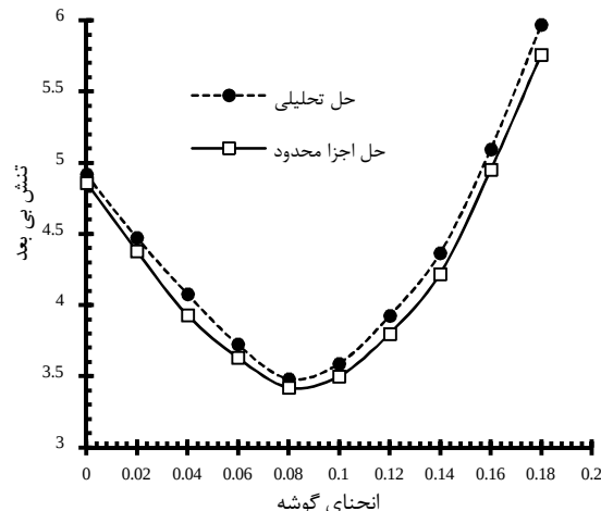
شکل 6 مقایسه تنش بی بعد اطراف گشودگی شبه مربعی برای ماده گرافیت/اپوکسی s[0 / 90] برحسب w از دو روش حل تحلیلی و اجزاء محدود
