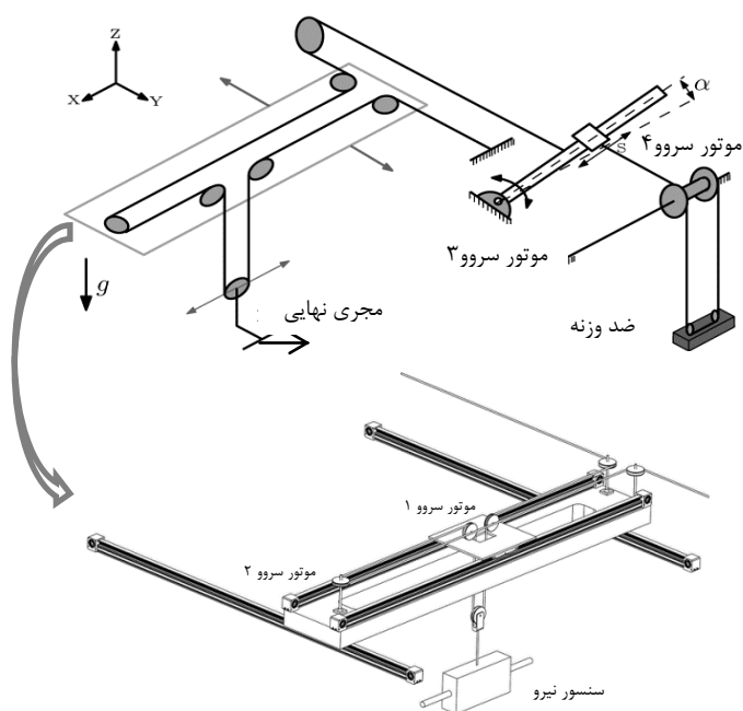
شکل ۱۷ کابل‌بندی جهت انتقال نیروی ضد وزنه به مجرى نهایی به همراه مدل سه بعدی مکانیزم جابجایی در راستای XY به کمک تسمه تایم
