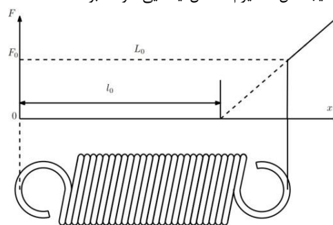
شکل ۳ مشخصات فنر
