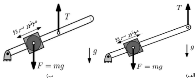
شکل ۱۴ مکانیزم ضد وزنه عمودی: (الف) نیروی T به انتهای بازو اعمال می‌شود و قابلیت تنظیم کمتر در نیروهای بالا دارد. (ب) نیروی T با فاصله از انتهای بازو وارد می‌شود و بازه‌ی نیرویی بیشتری را پوشش می‌دهد
