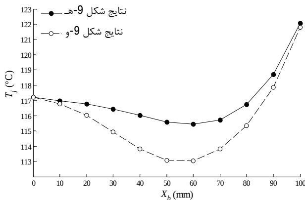
شکل 11 دمای بیشینه برای چیدمان شکل 9-ه و شکل 9-و با تغییر X_b
