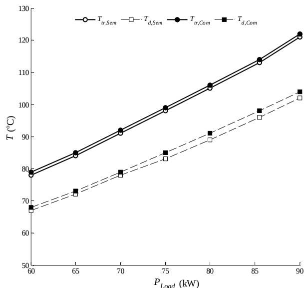
شکل 8 مقایسه بین نتایج حاصل از شبیه‌سازی و نرم‌افزار سیمپل
