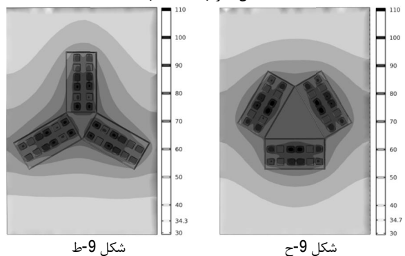
شکل 13 توزیع دمایی در چیدمان‌های انتخابی (جدول 8)
