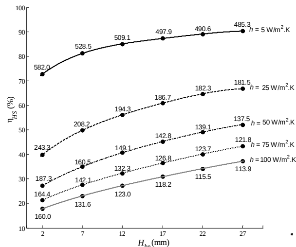
شکل 17 تغییر ضخامت پایه گرمابری
