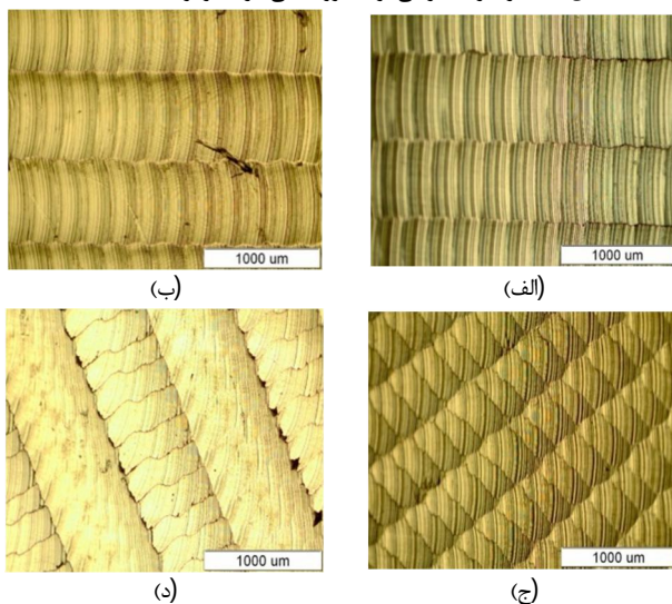
شکل 10 مقایسه بافت سطحی استراتژی‌ها در آزمایش دوم (الف خطوط موازی ب) آفست سه بعدی ج) مارپیچ د) شعاعی
