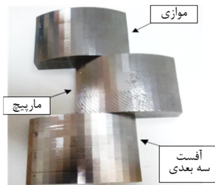
شکل 3 الف) شماتیک مناطق مربوط به هر آزمایش روی نمونه‌های محدب ب) نمونه‌های ماشینکاری شده توسط استراتژی مختلف
