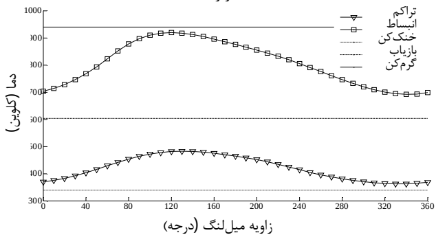
شکل 8 منحنی تغییرات دما در 4/14 مگاپاسکال و 41/67 هرتز
