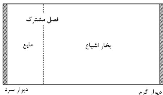
شکل 1 شرایط مسئله‌ی استفان
