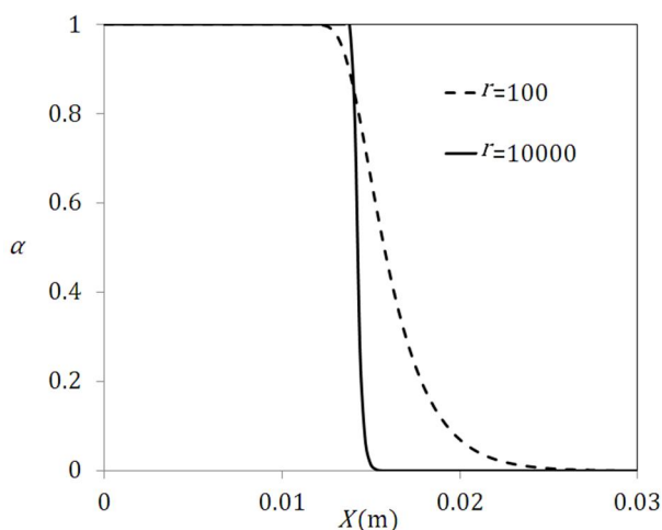
شکل 3 توزیع حجم سیال در زمان t=100\text{sec} در مسئله‌ی استفان، تیز شدن فصل مشترک با افزایش ضریب شدت انتقال جرم
